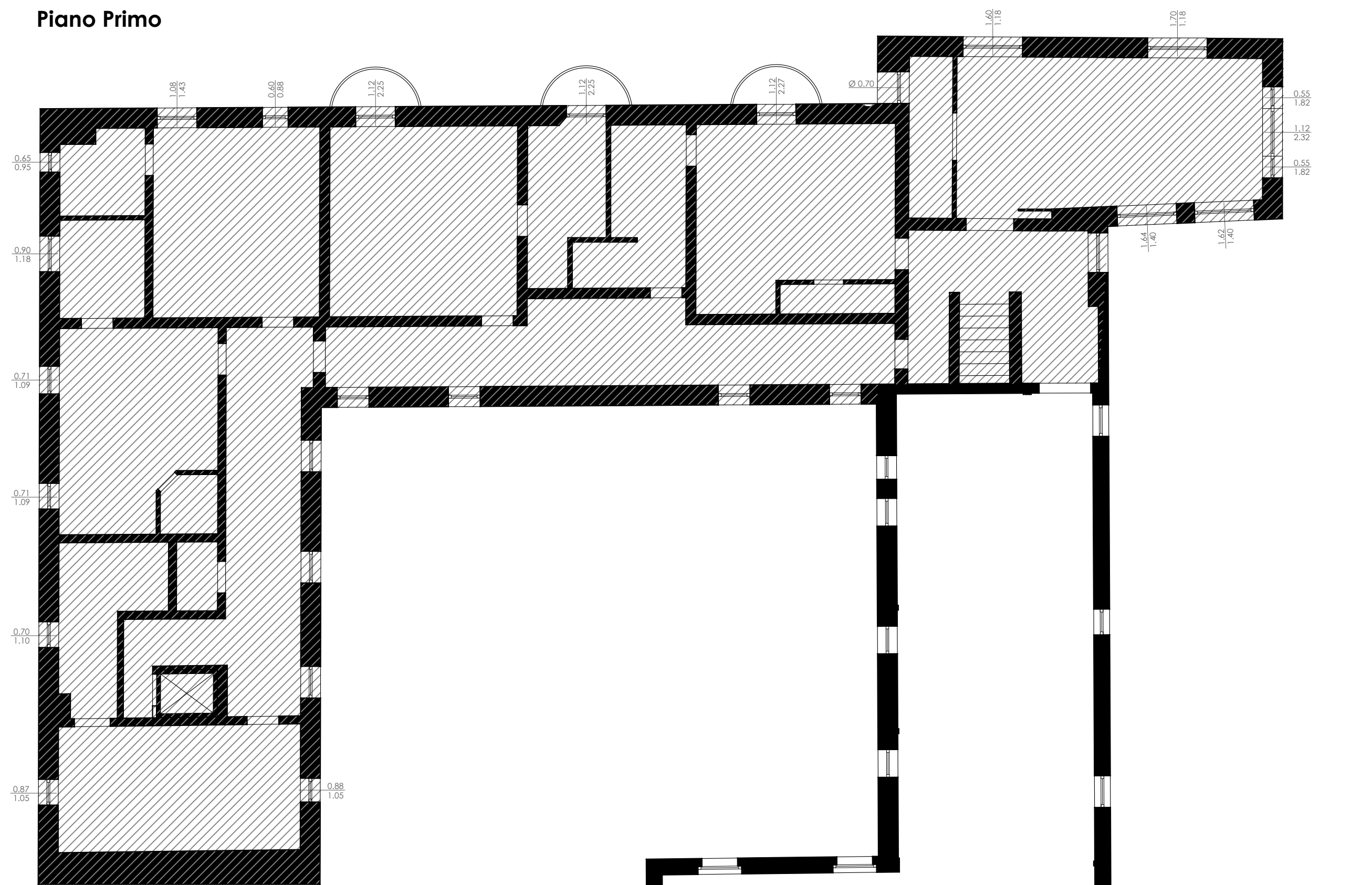
Piano Primo
